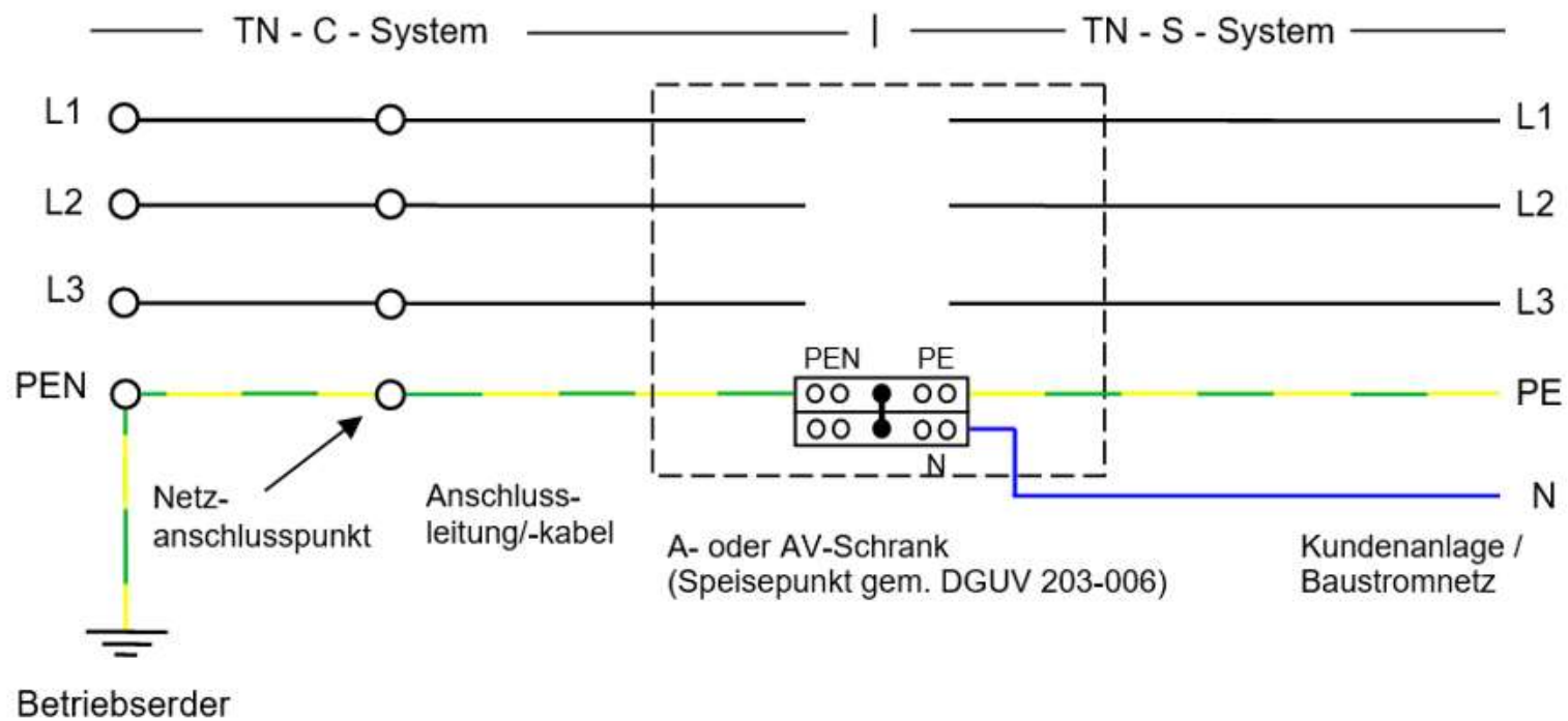
Abbildung 7 - Anschlussmöglichkeiten am Beispiel des TN-C-Systems
