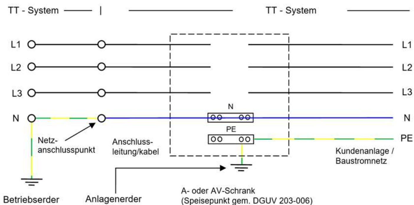
Abbildung 8 - Anschlussmöglichkeiten am Beispiel des TT-Systems
